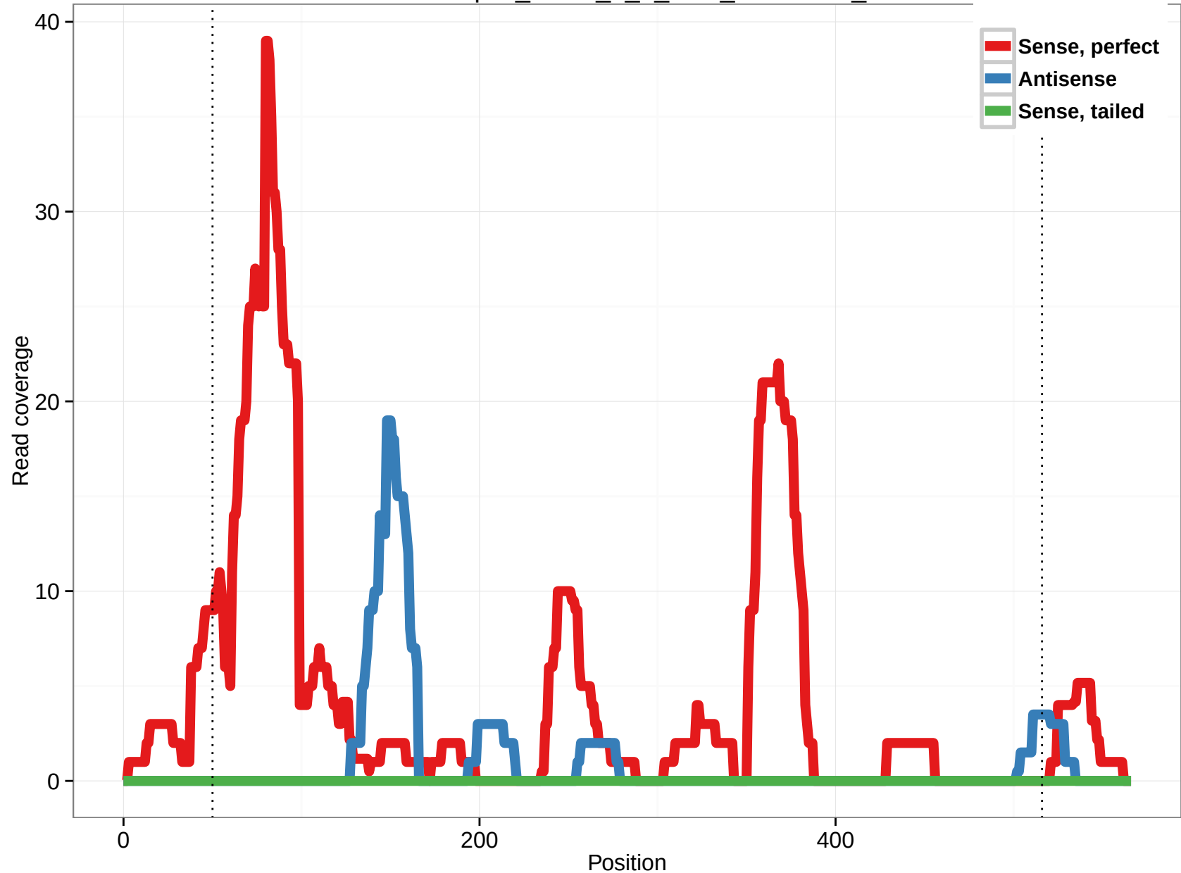
uc001aqo.2_intron_6_0_chr1_10002841_r
