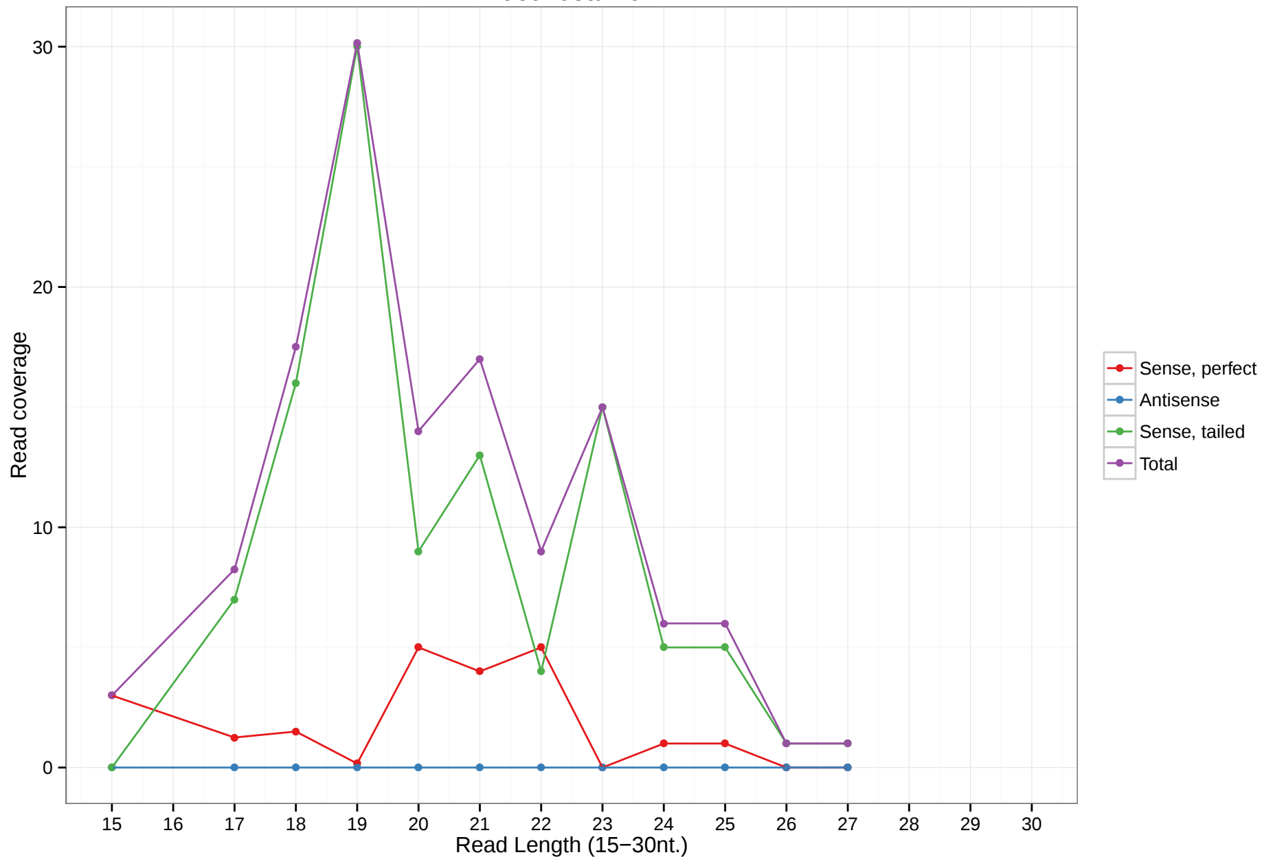
uc010oaf.10
