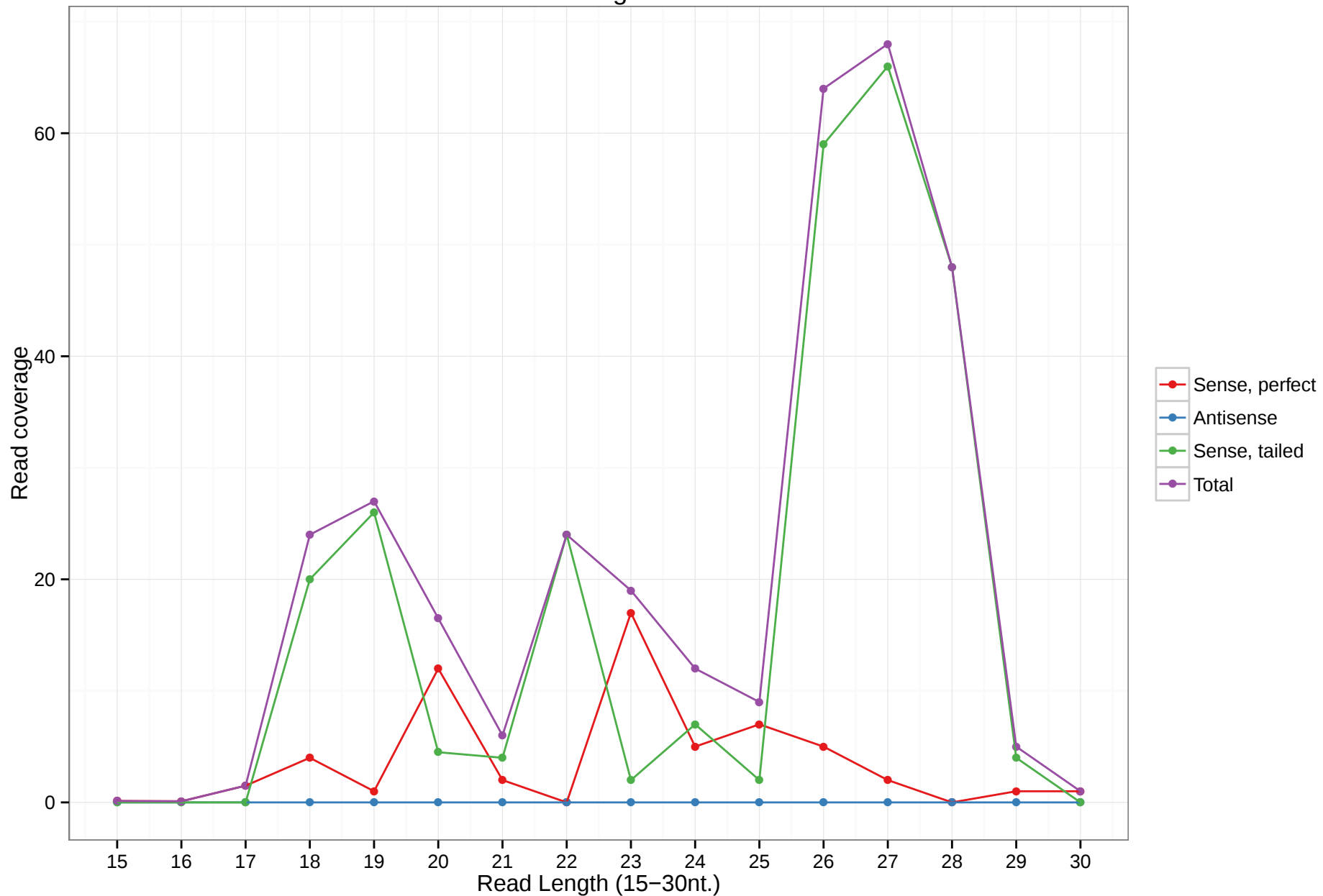
uc010lgo.1
