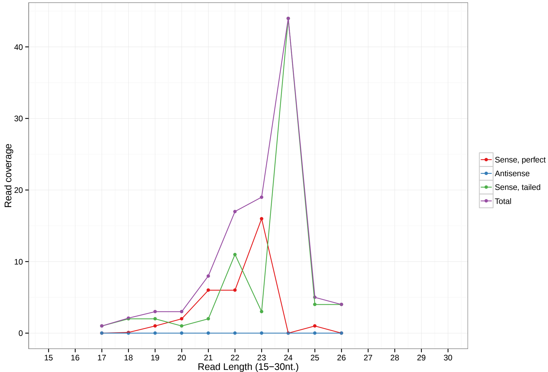
uc010eei.27
