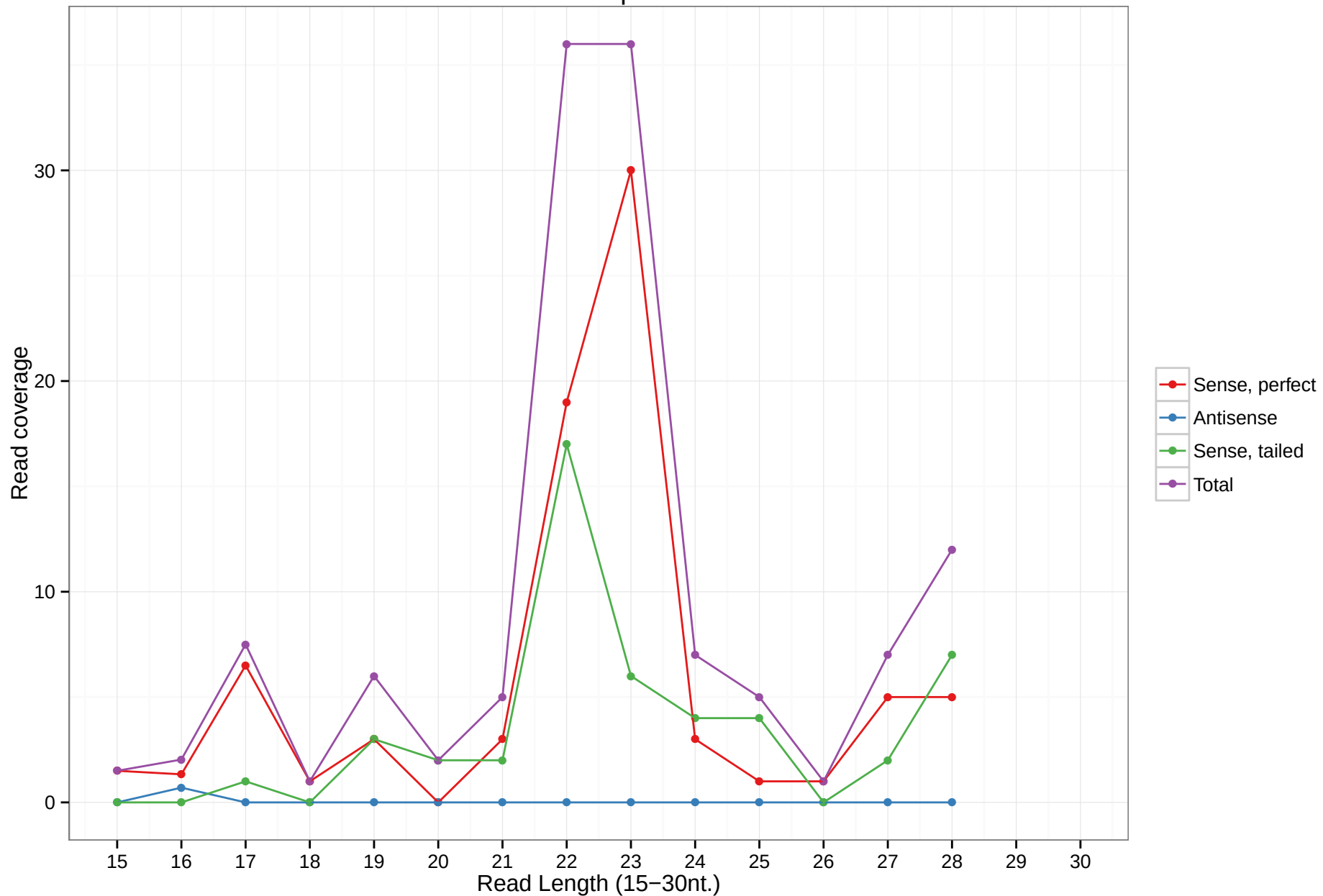
uc009zpl.1
