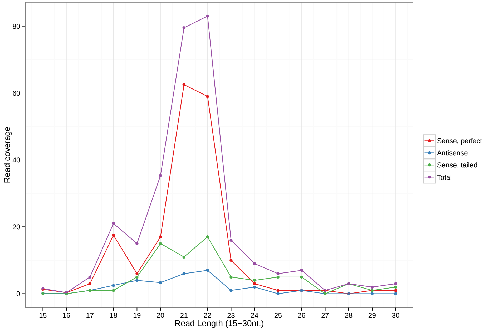
uc003zwe.11
