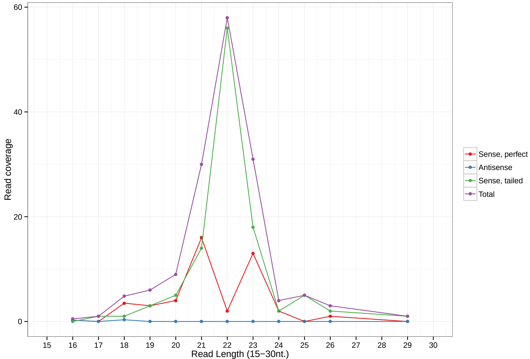
uc003cum.7
