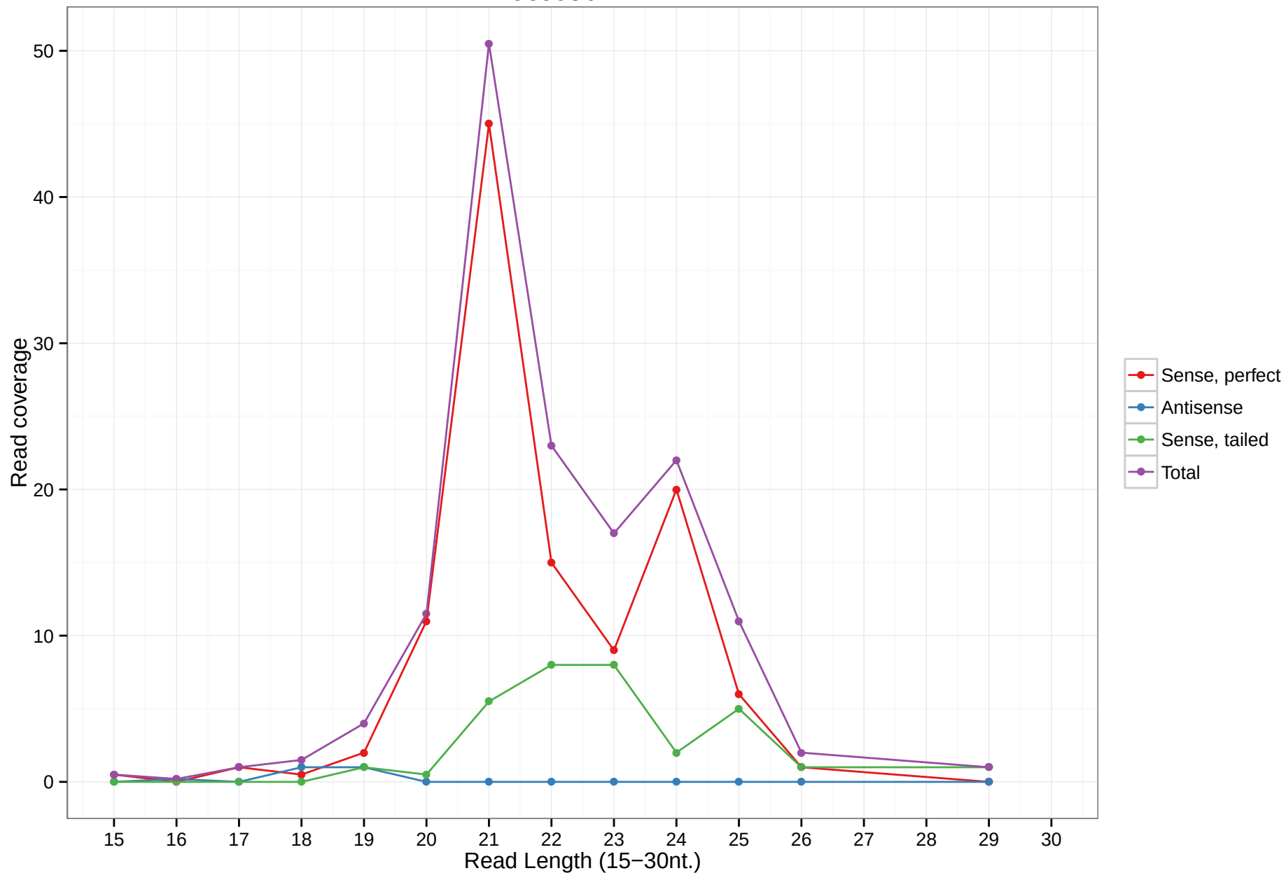
uc003bmk.7
