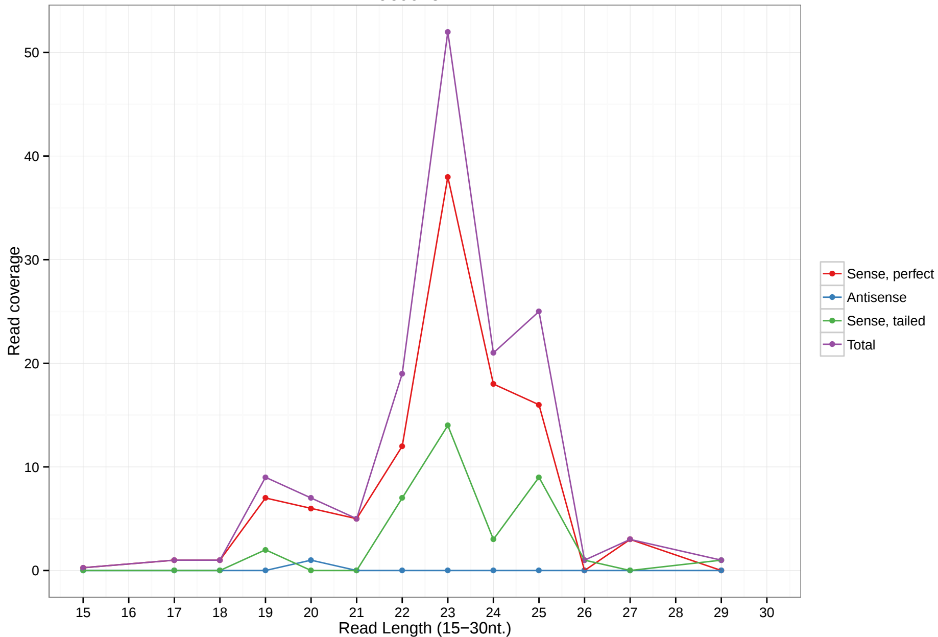
uc001okr.2
