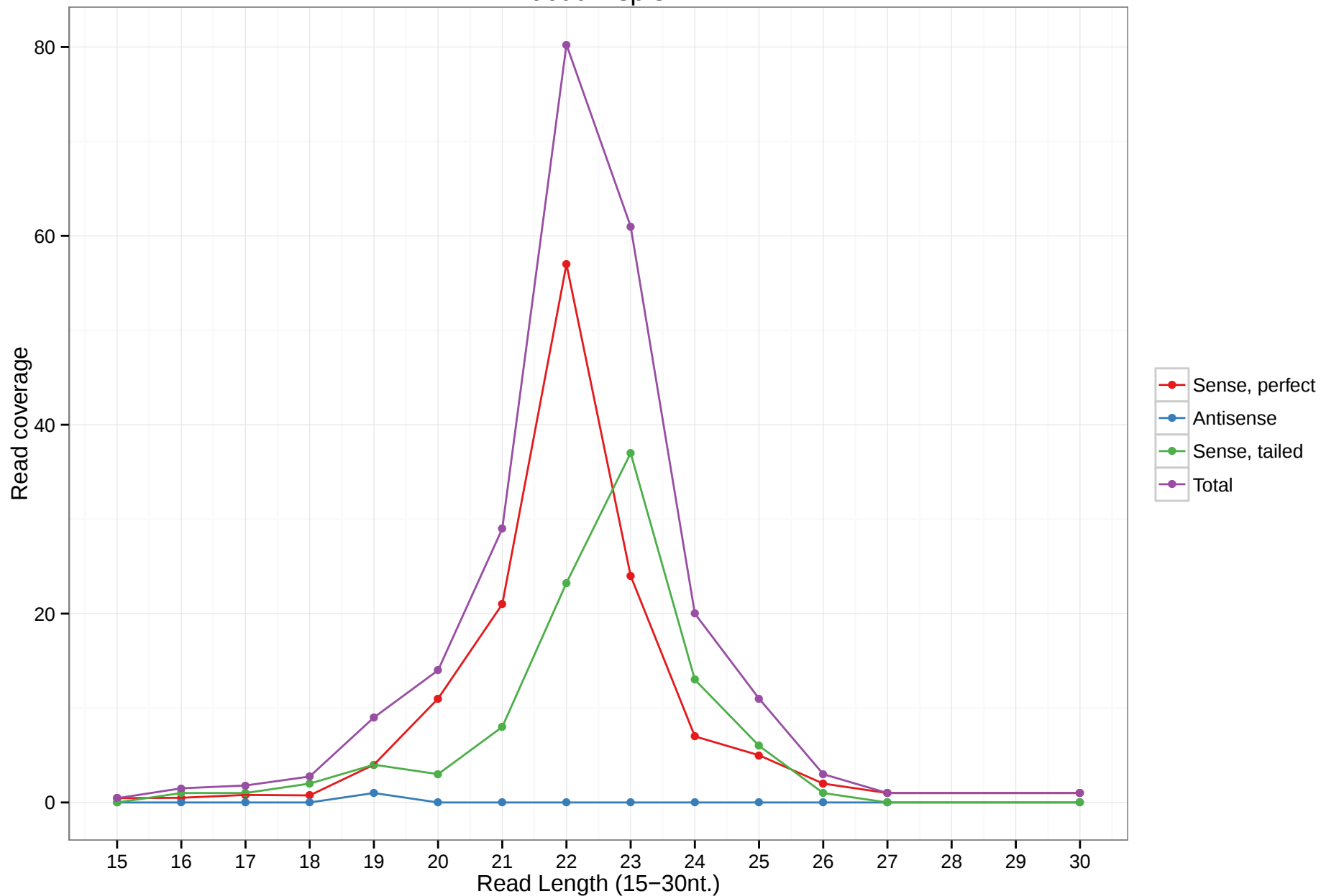
uc001ksp.8
