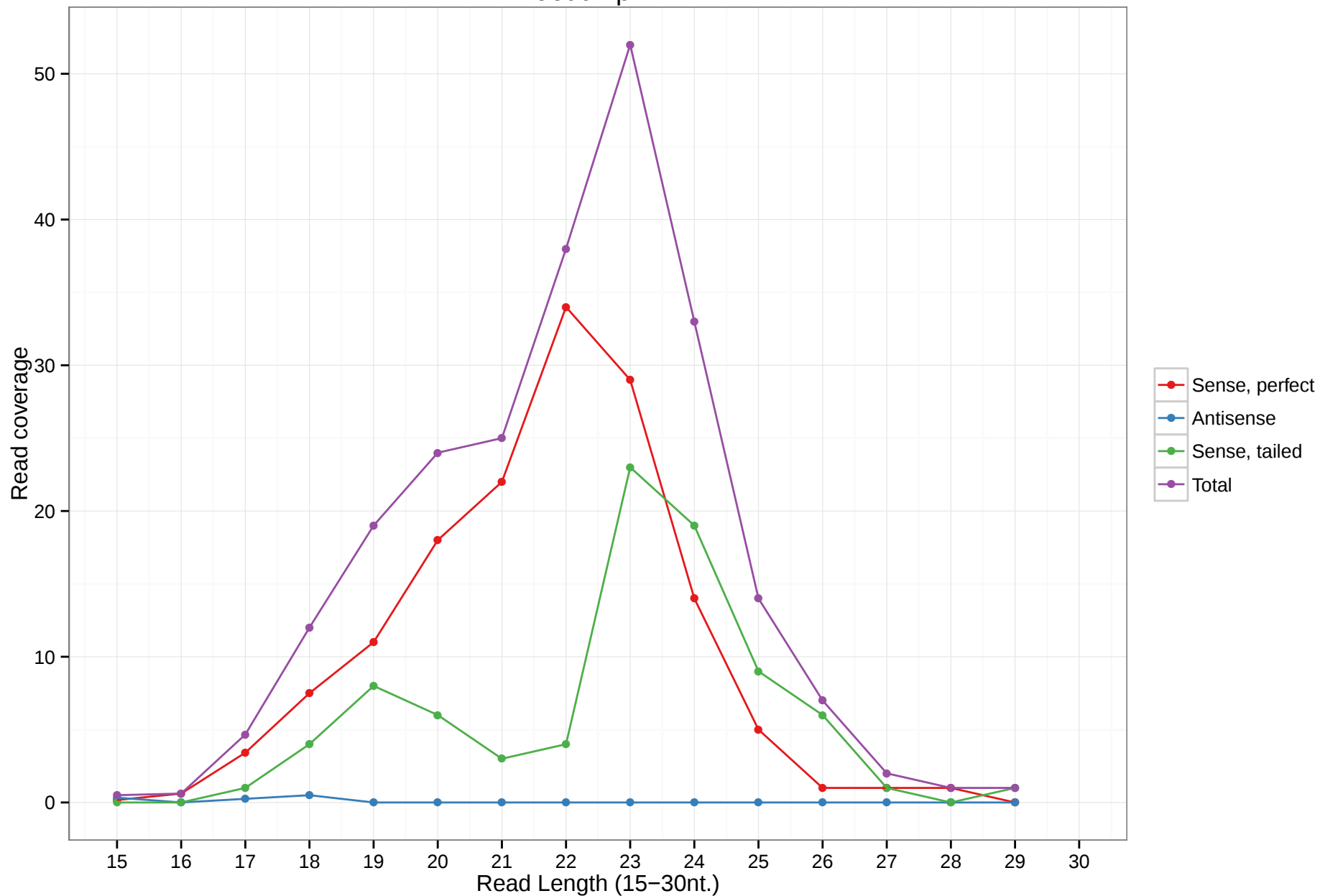
uc001fpr.2
