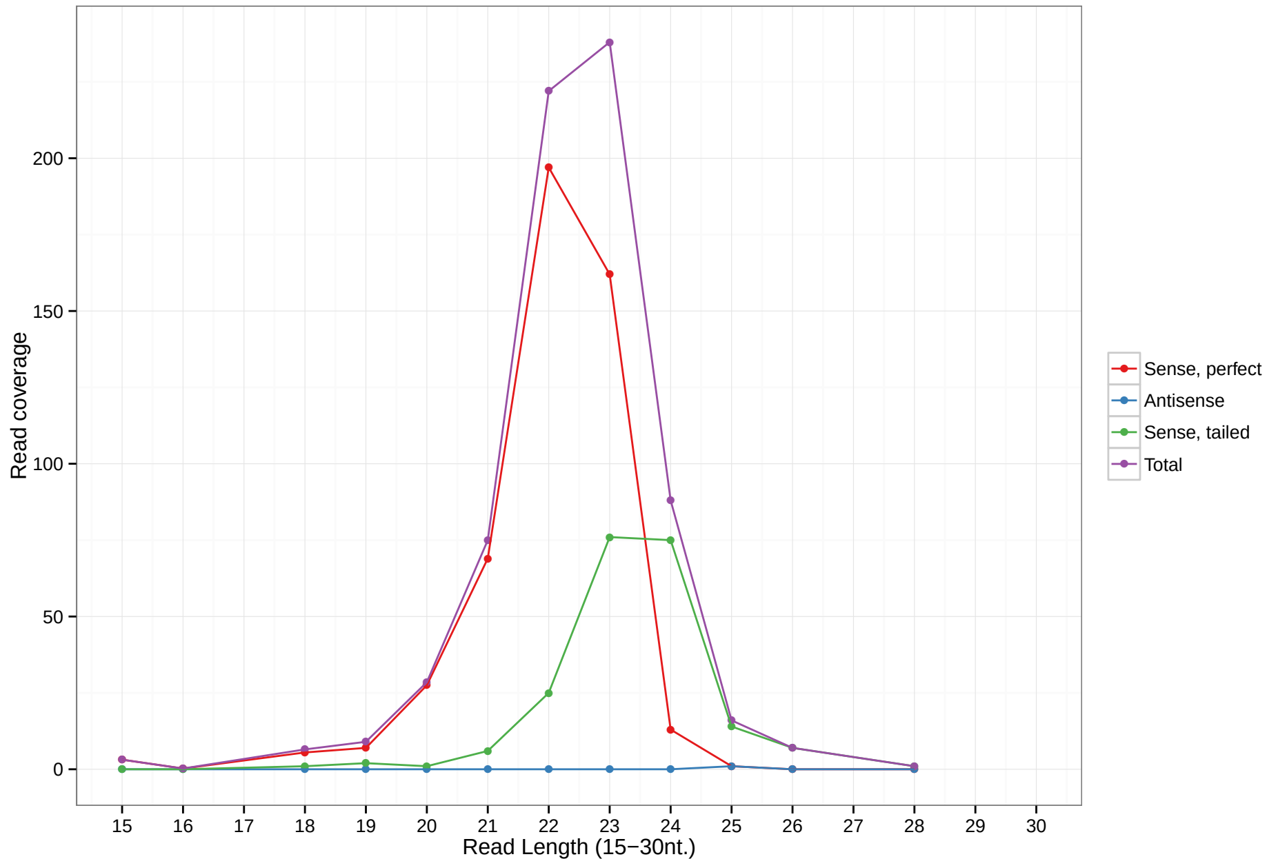
uc001eto.1
