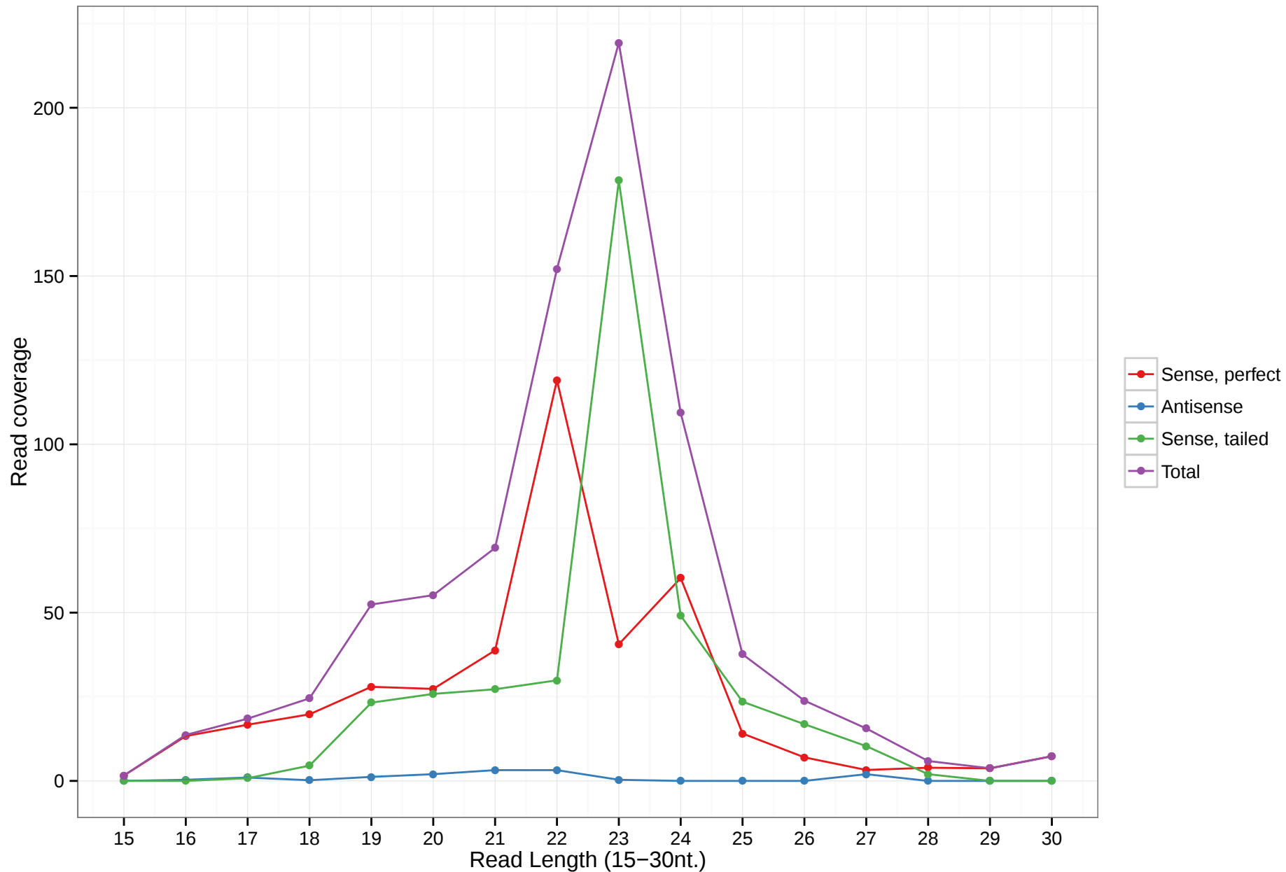
hsa-mir-7111
