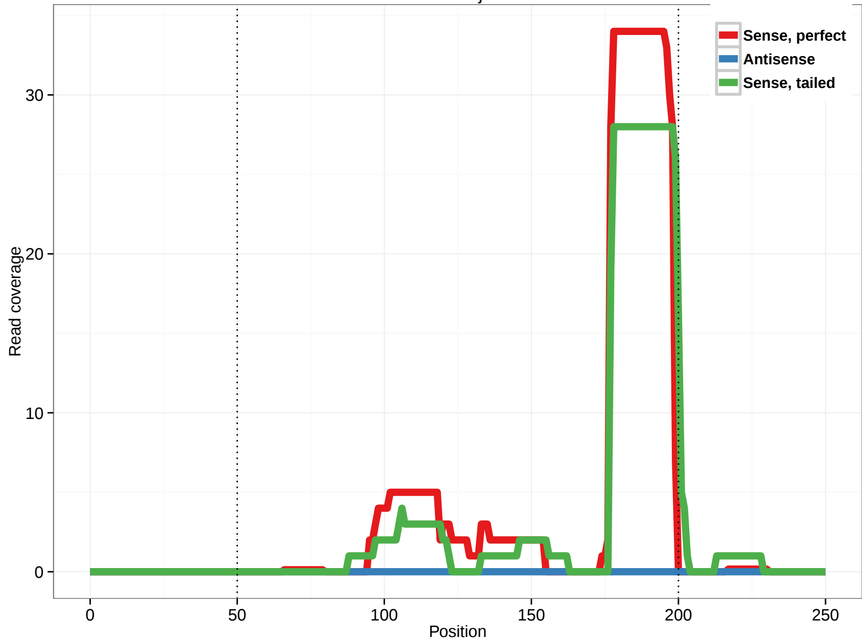
uc010ncj.16
