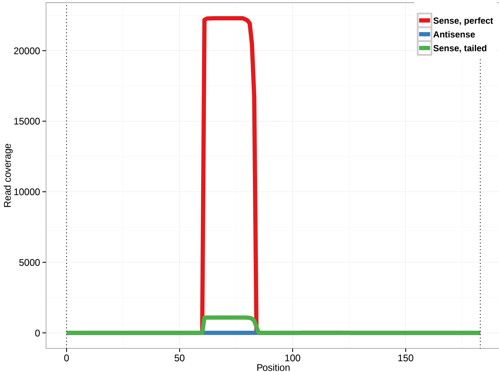
mir-315
