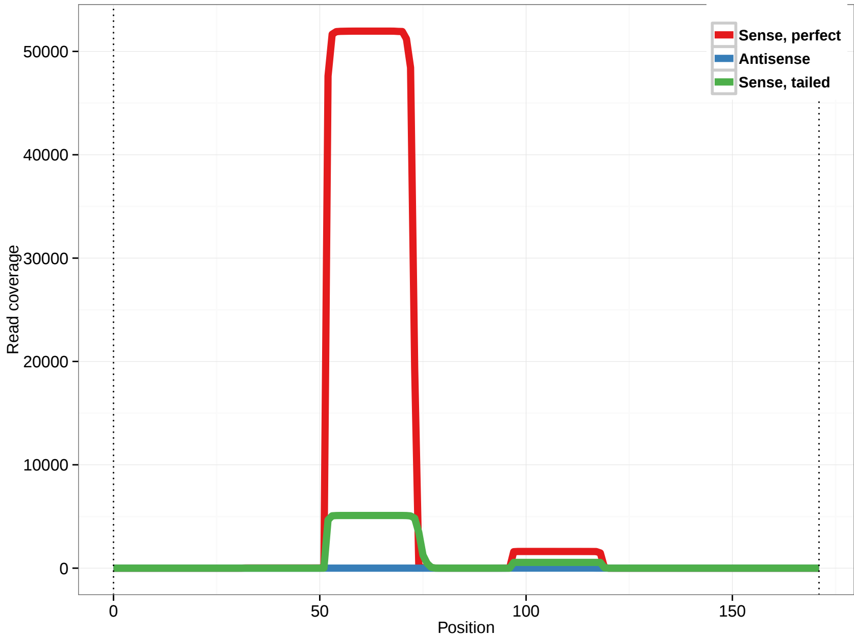
mir-306
