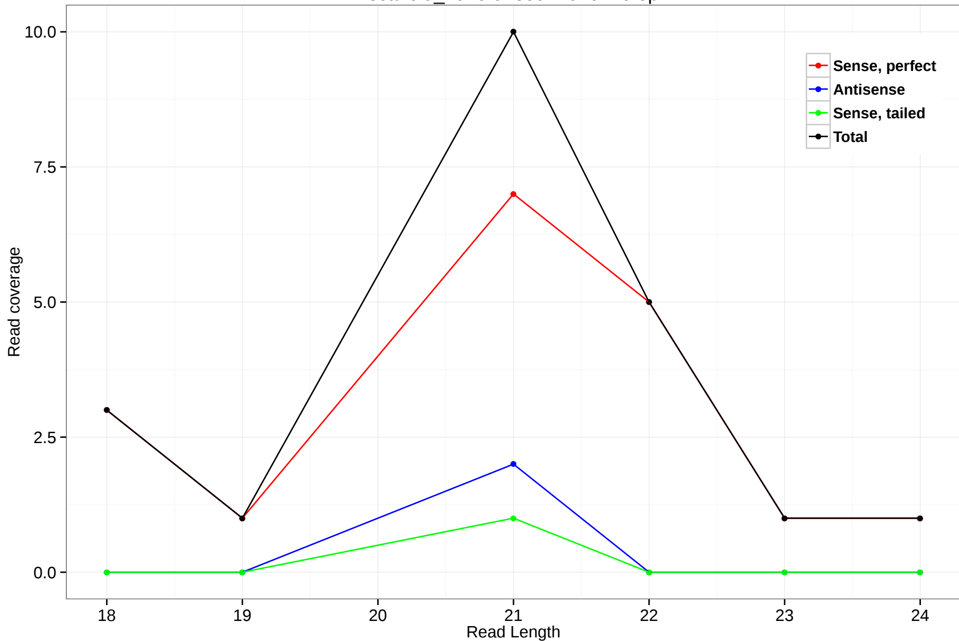
scaffold_4929:928591-929479.3p
