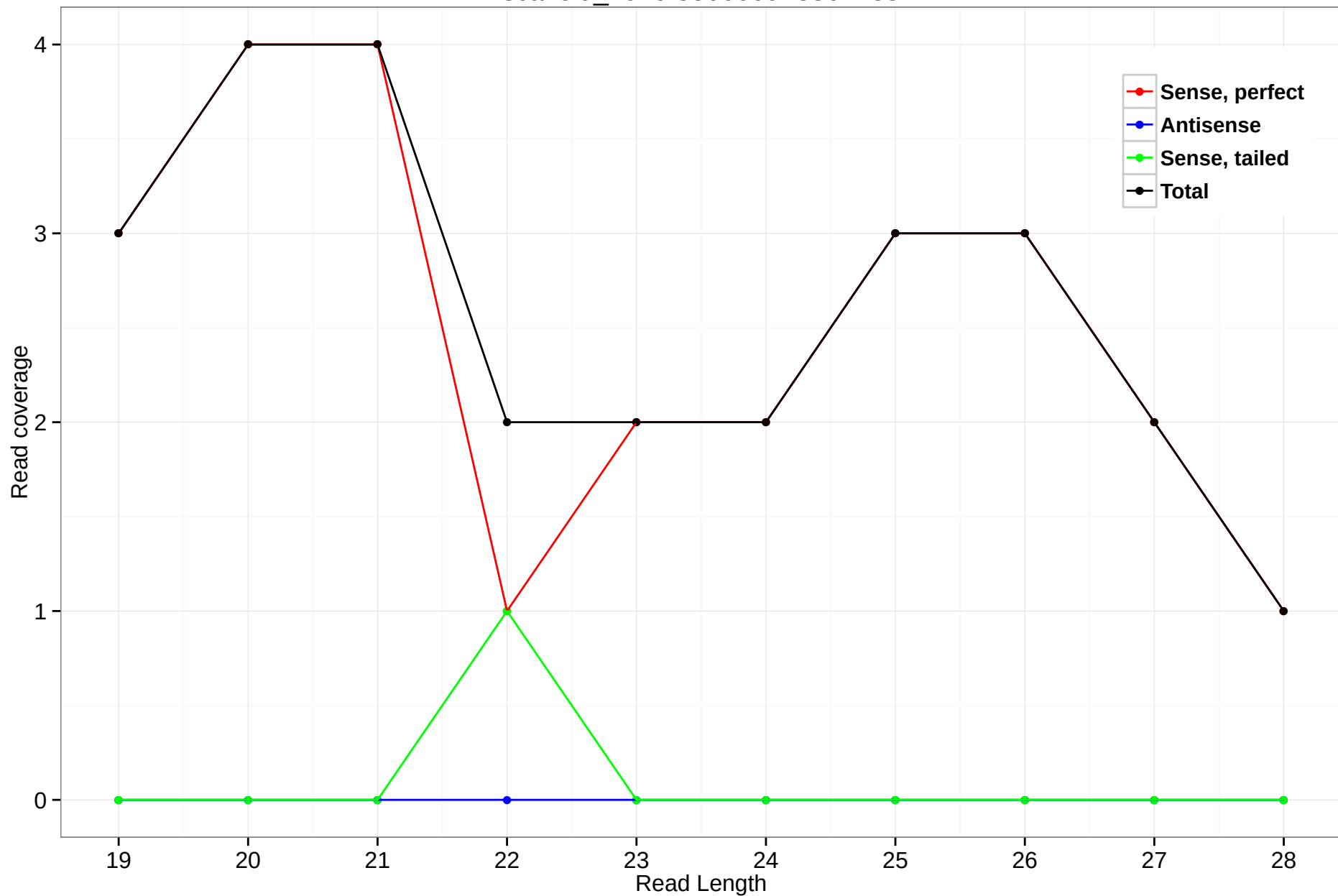
scaffold_4929:8366669-8367185
