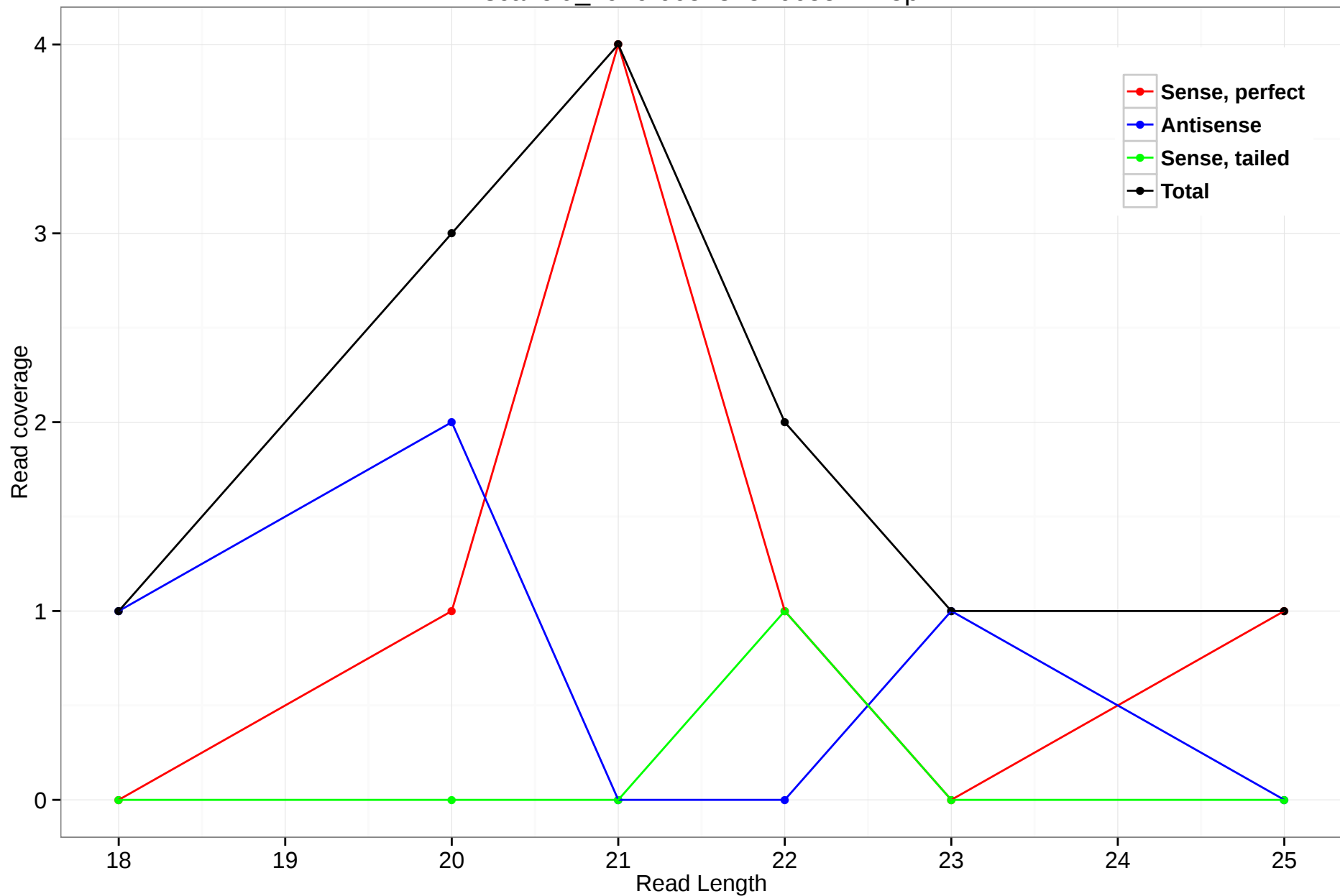
scaffold_4929:6652375-6655214.5p
