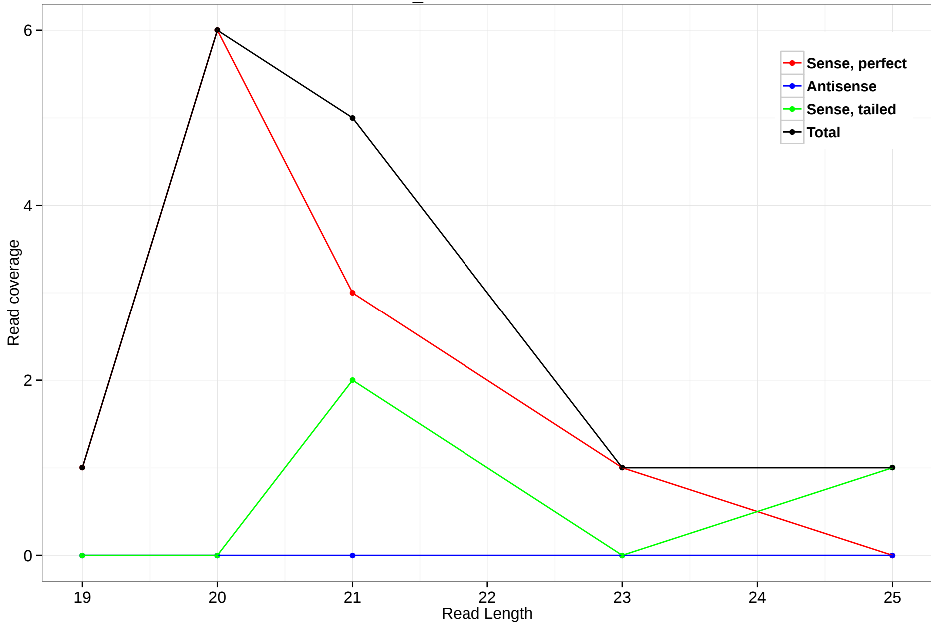
scaffold_4929:2929634-2929914
