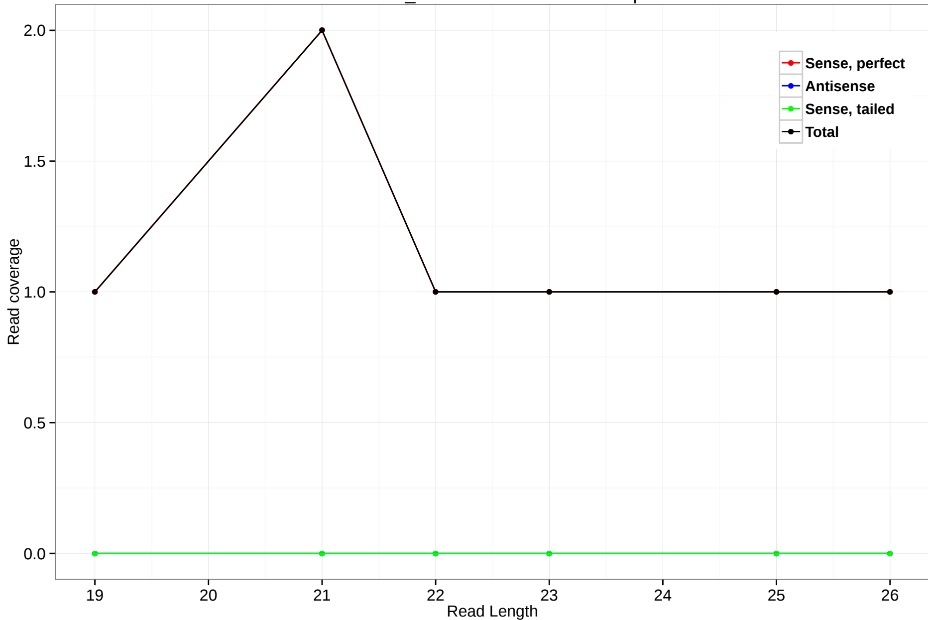
scaffold_4845:9389127-9389819.3p
