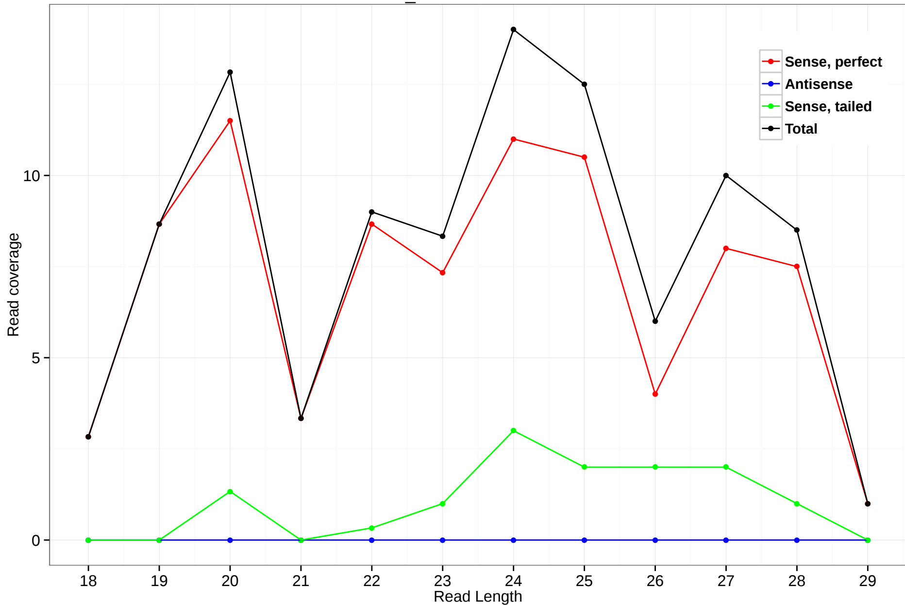
scaffold_4845:7818099-7818377
