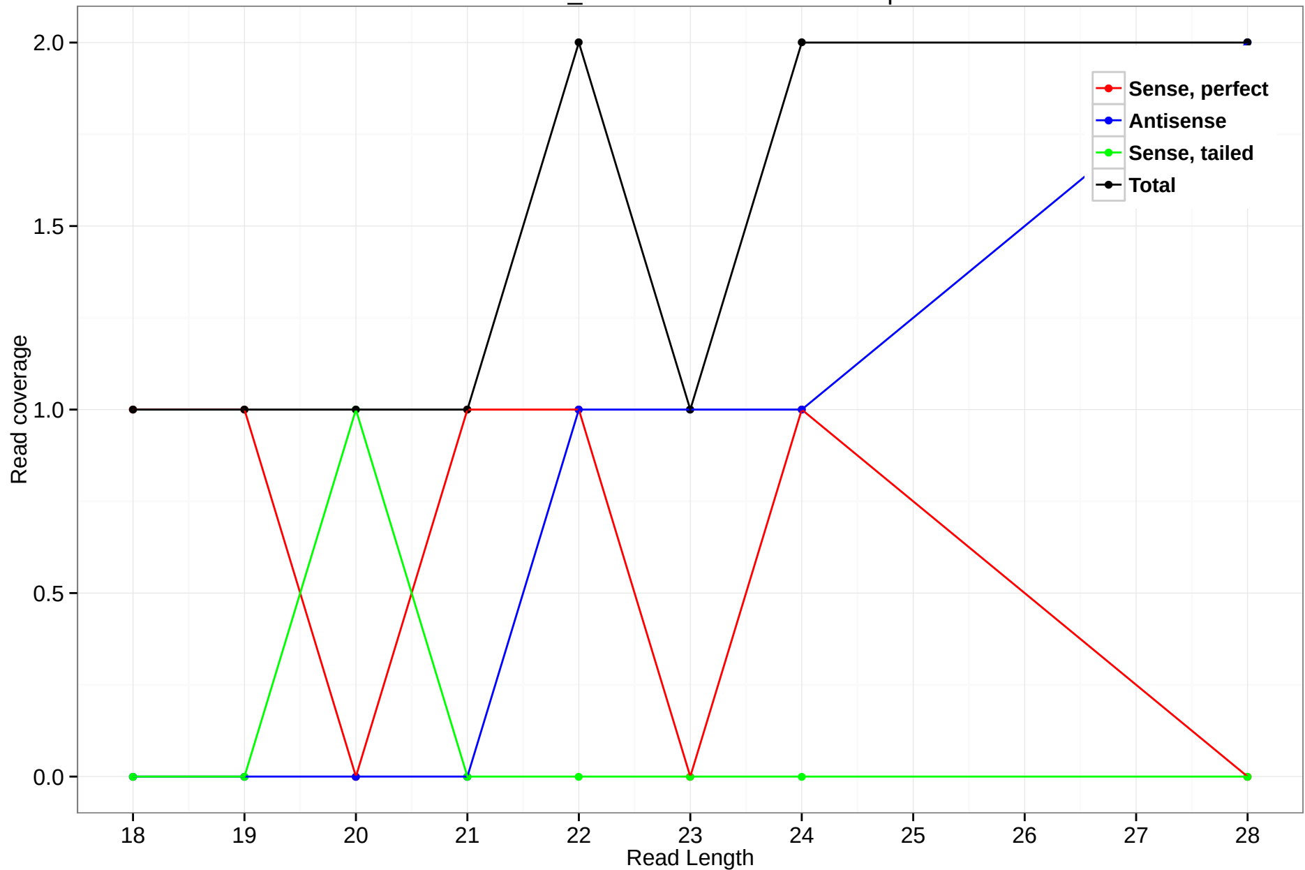
scaffold_4845:3639178-3639801.5p
