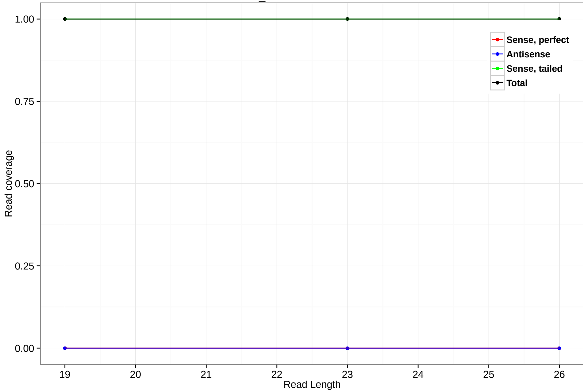
scaffold_4770:14387501-14387669
