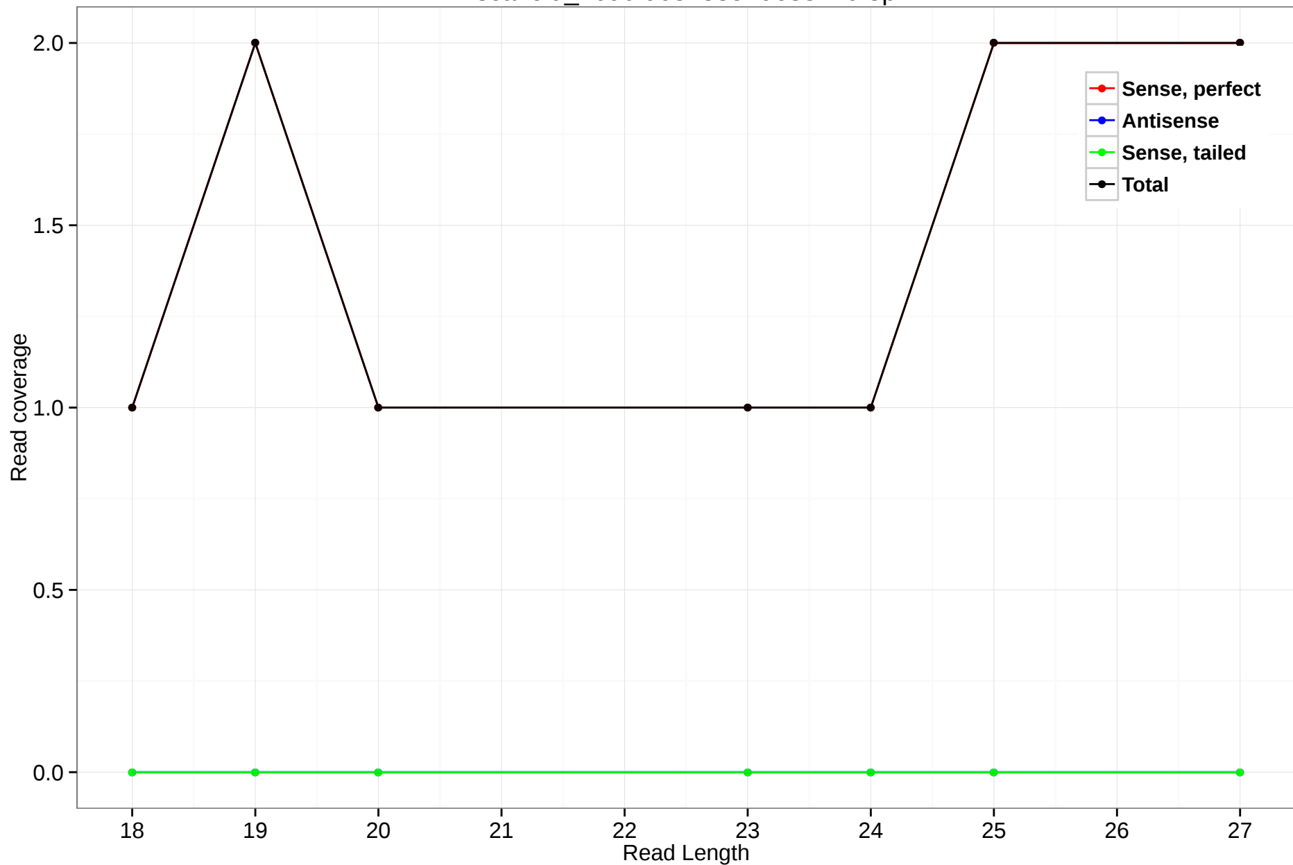
scaffold_4690:9631335-9638219.3p
