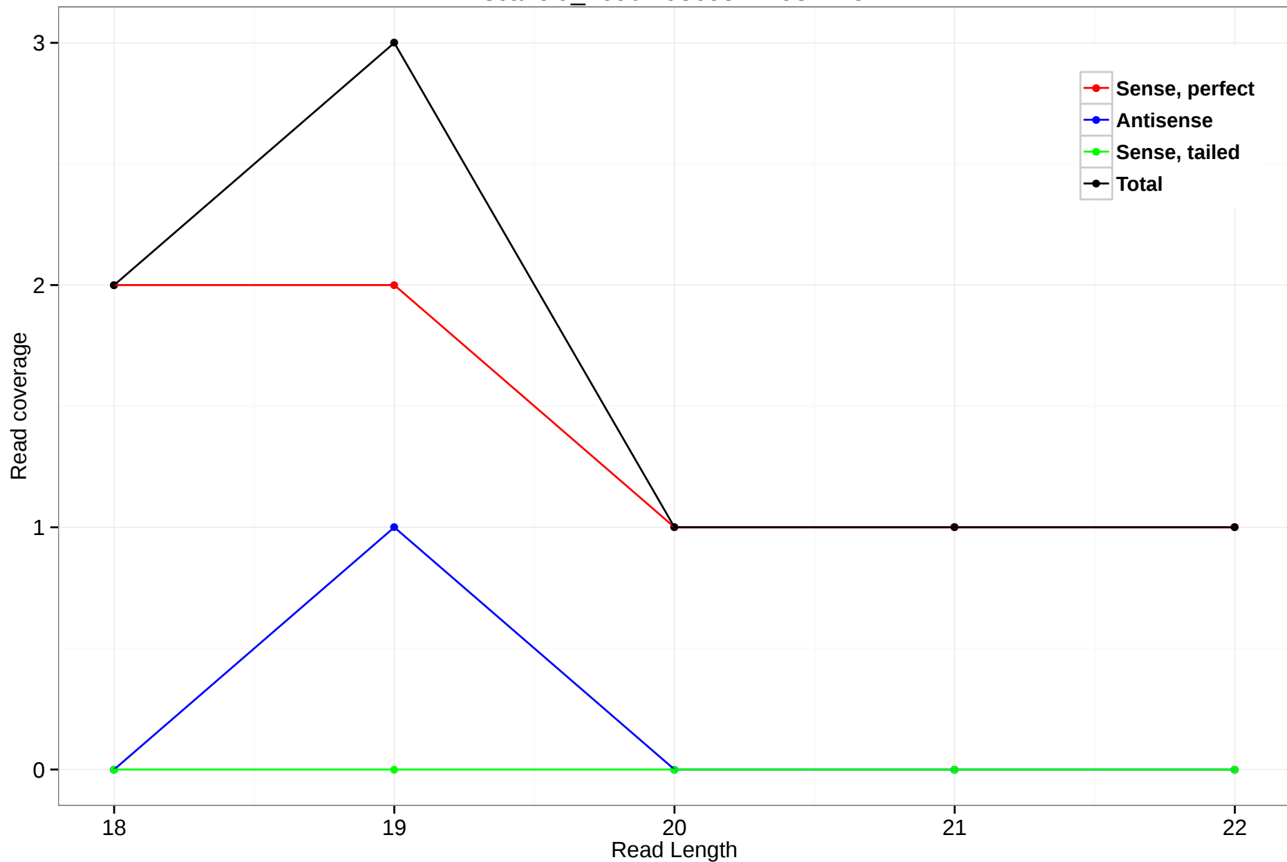
scaffold_4690:2936951-2937215
