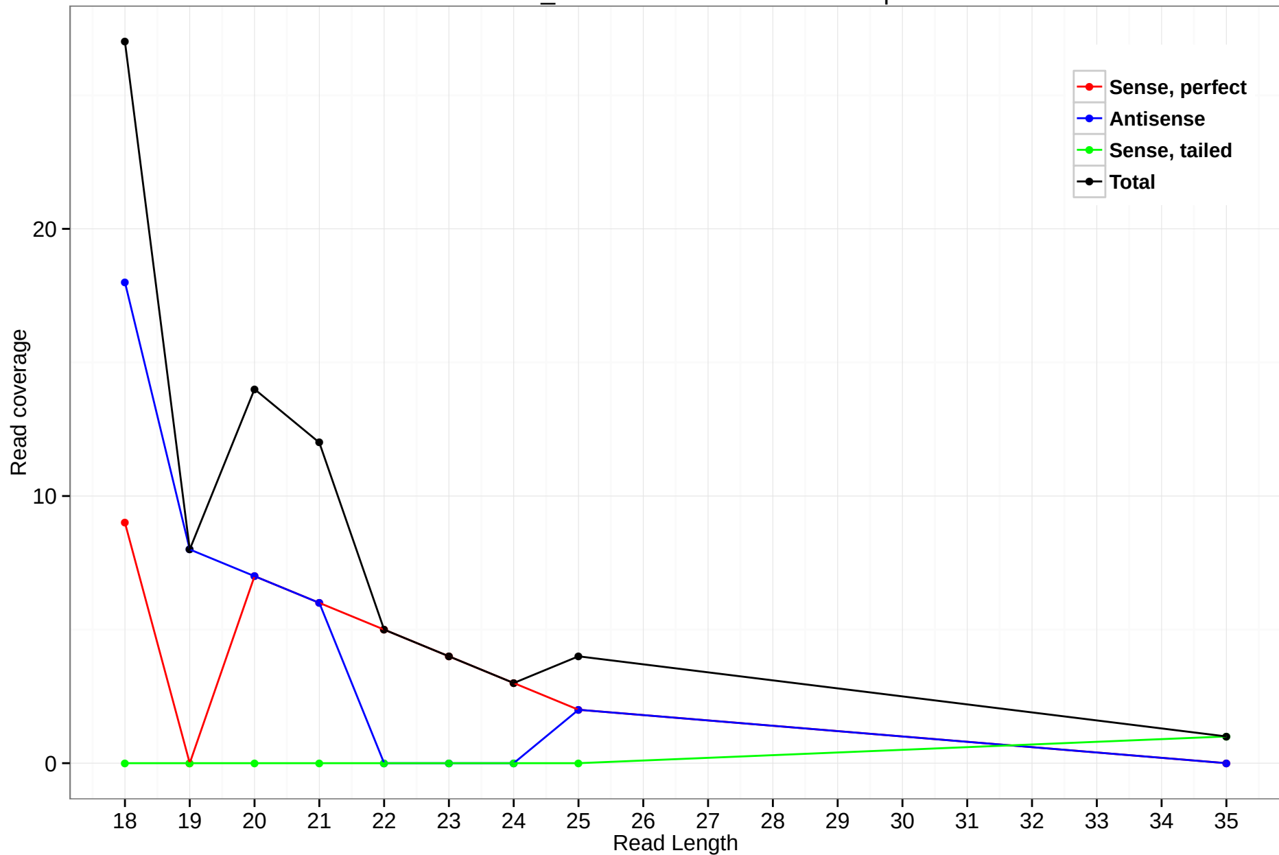
scaffold_4690:14988647-14993724.3p
