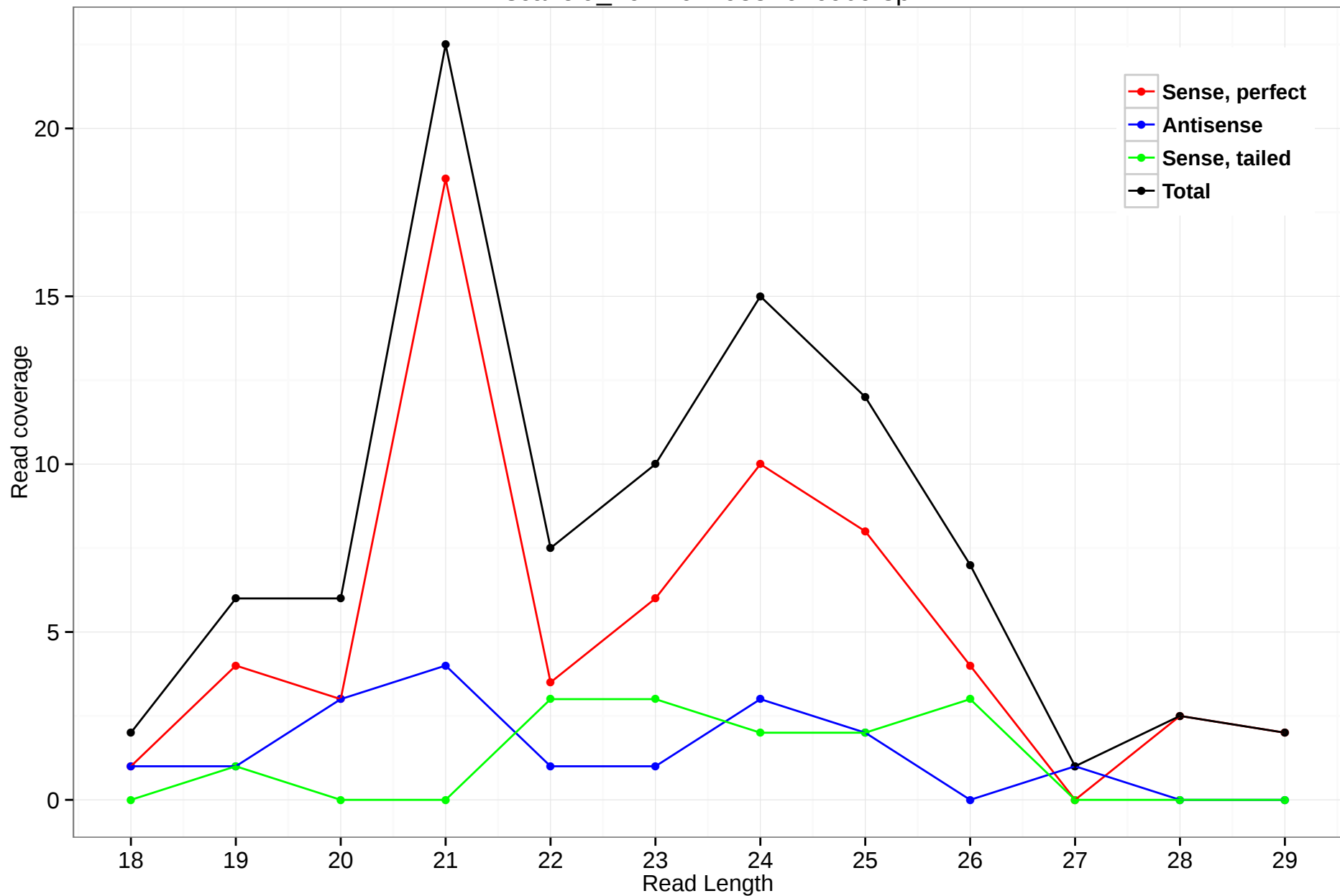
scaffold_4644:614955-616909.3p
