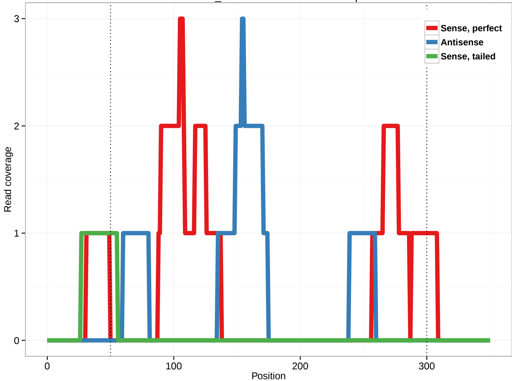
scaffold_4929:8517479-8518087.5p
