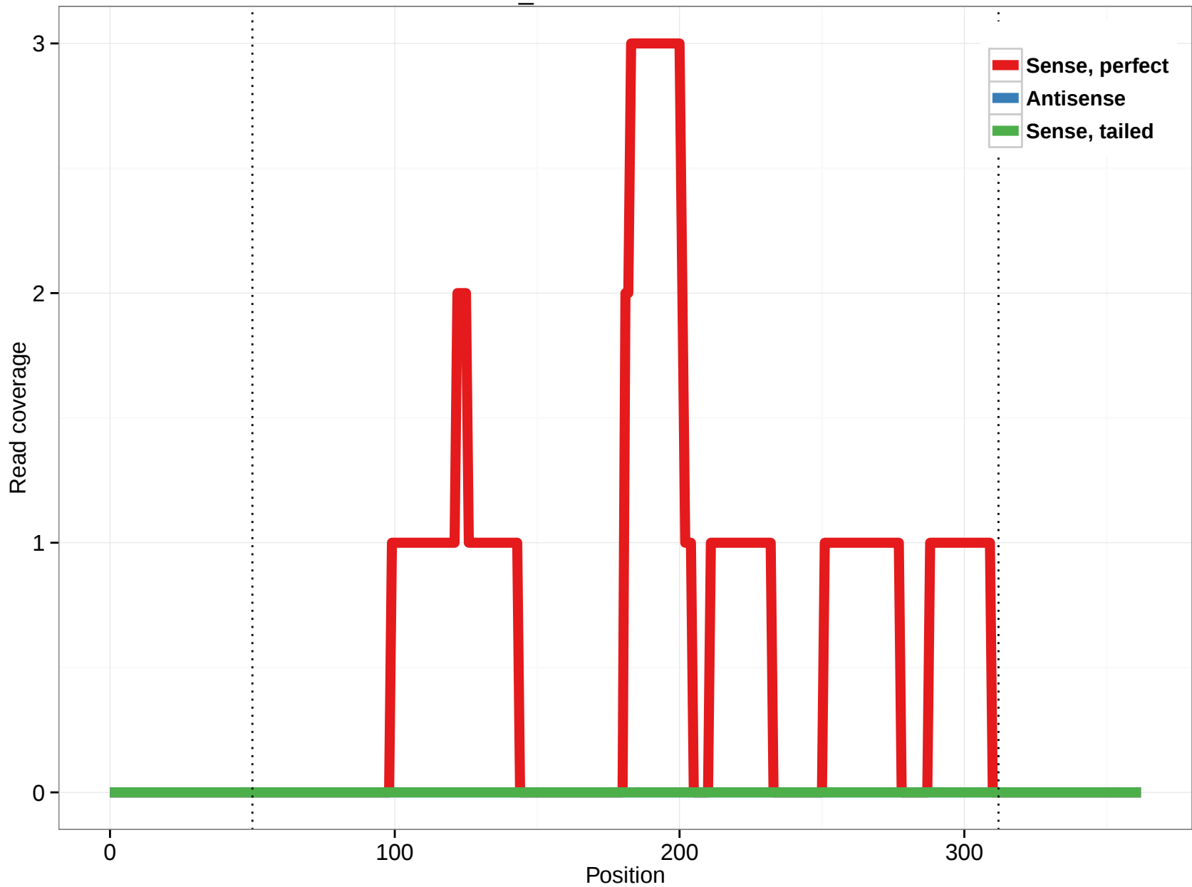
scaffold_4845:8717713-8718075
