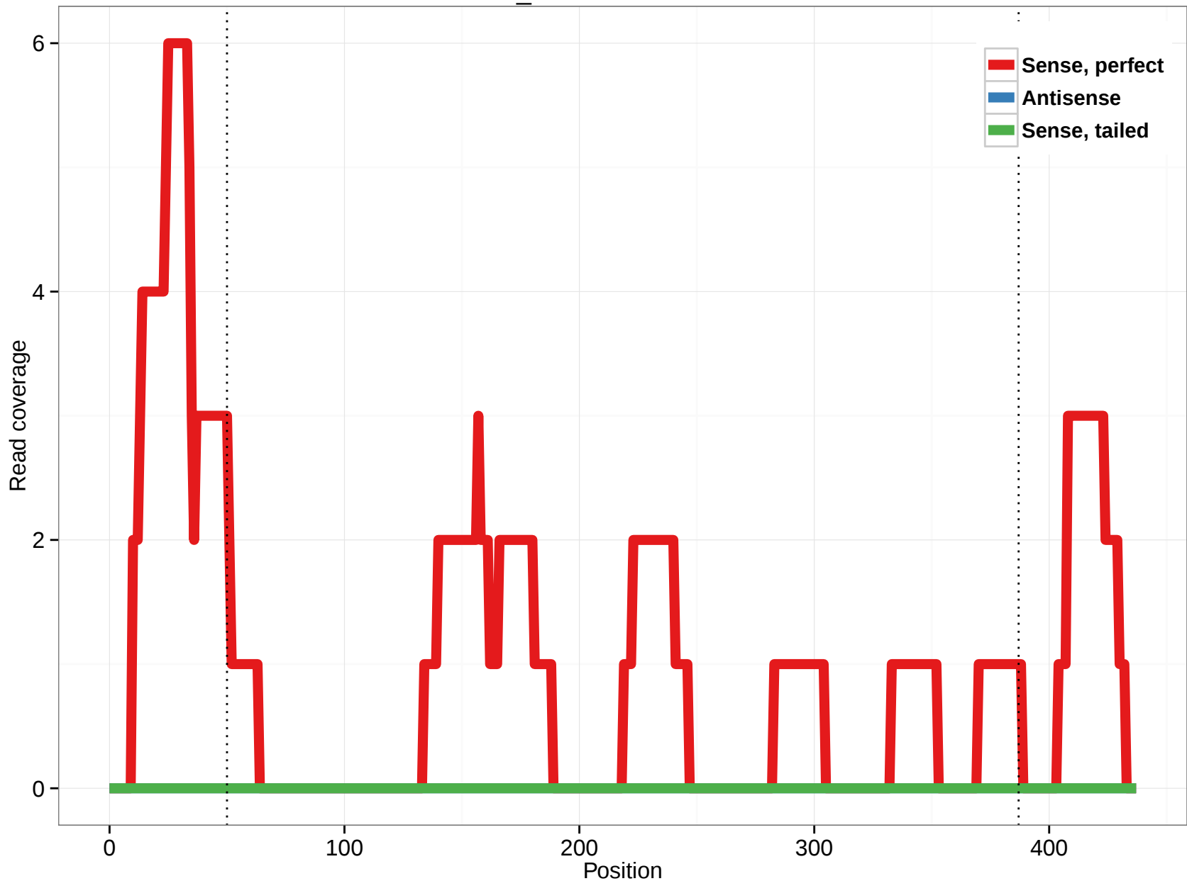
scaffold_4820:3898919-3899356
