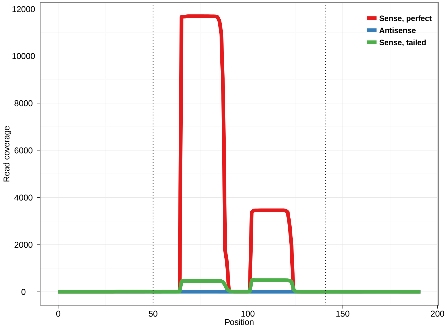
dme-mir-992
