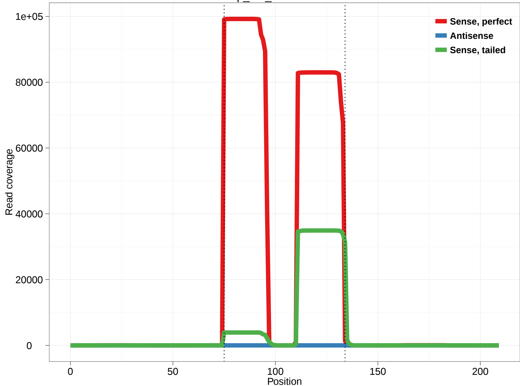
Lerp_in6_dme-mir-1012
