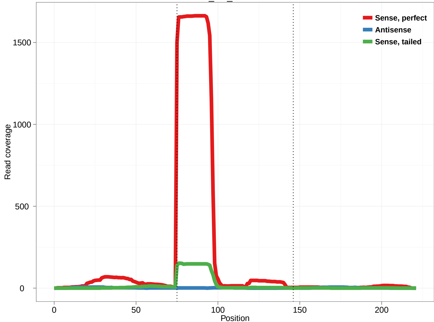
CG7927_in2_dme-mir-2501
