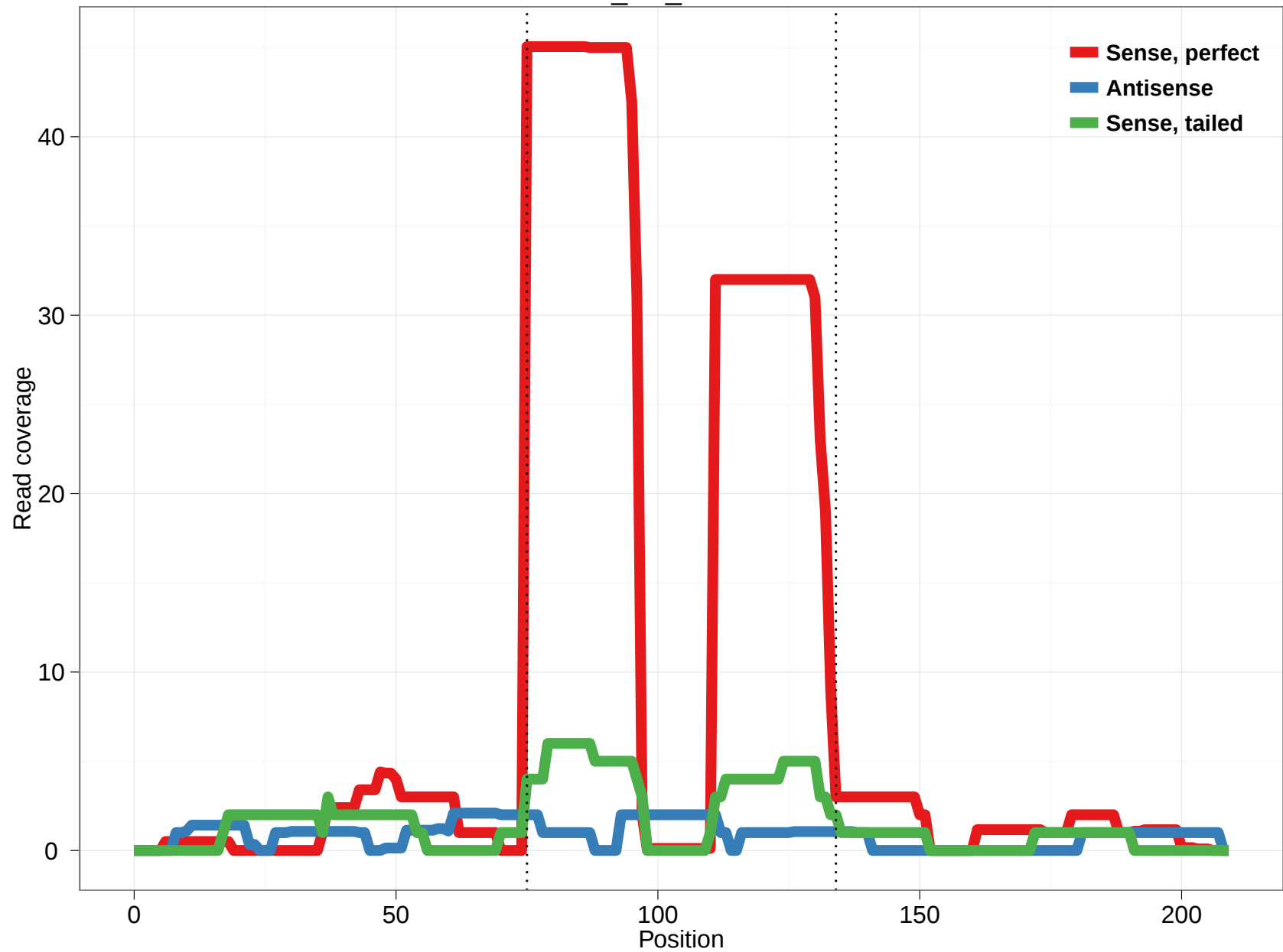
CG32704_in1_dme-mir-4916
