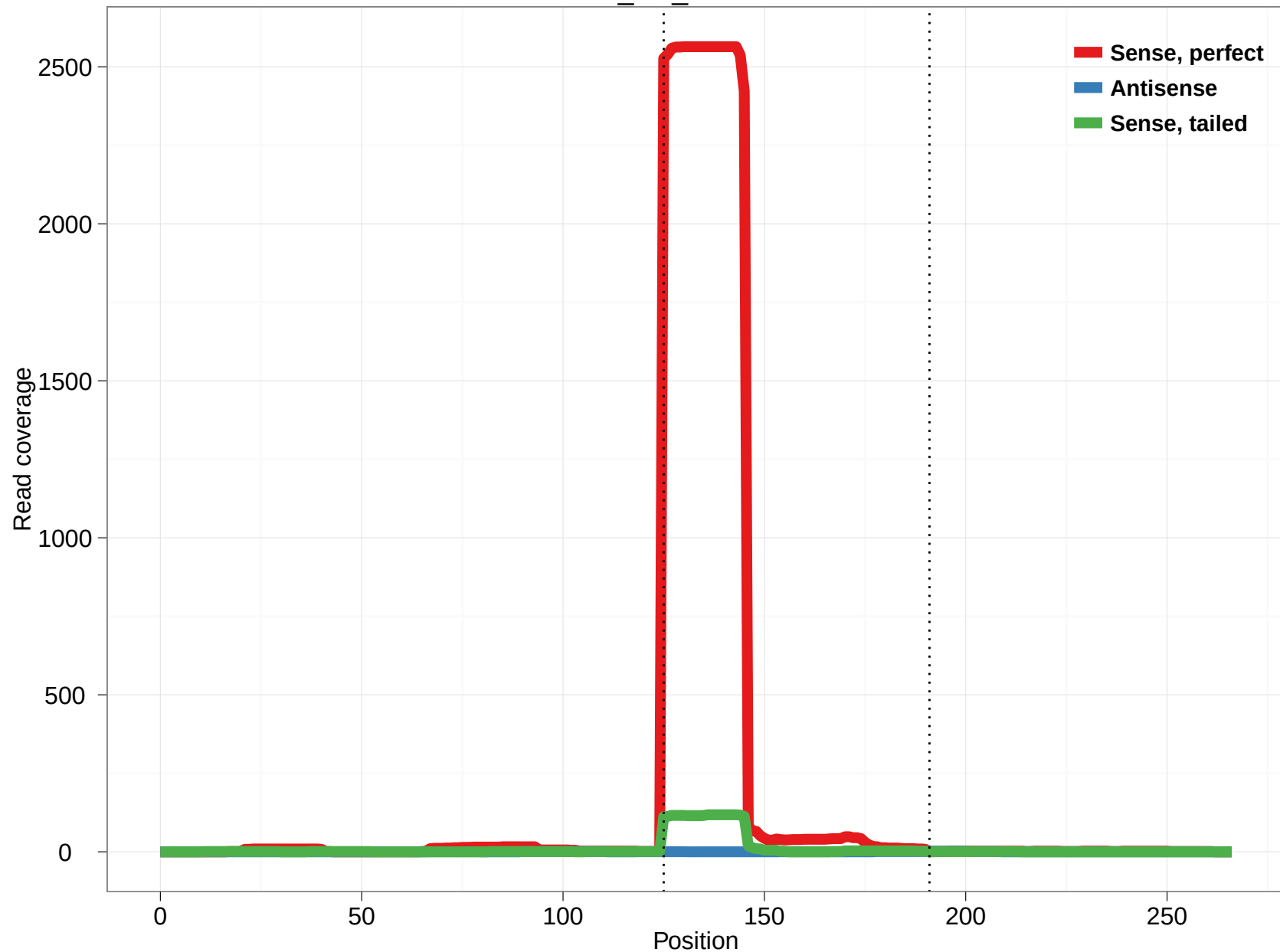
CG3225_in2_dme-mir-4910
