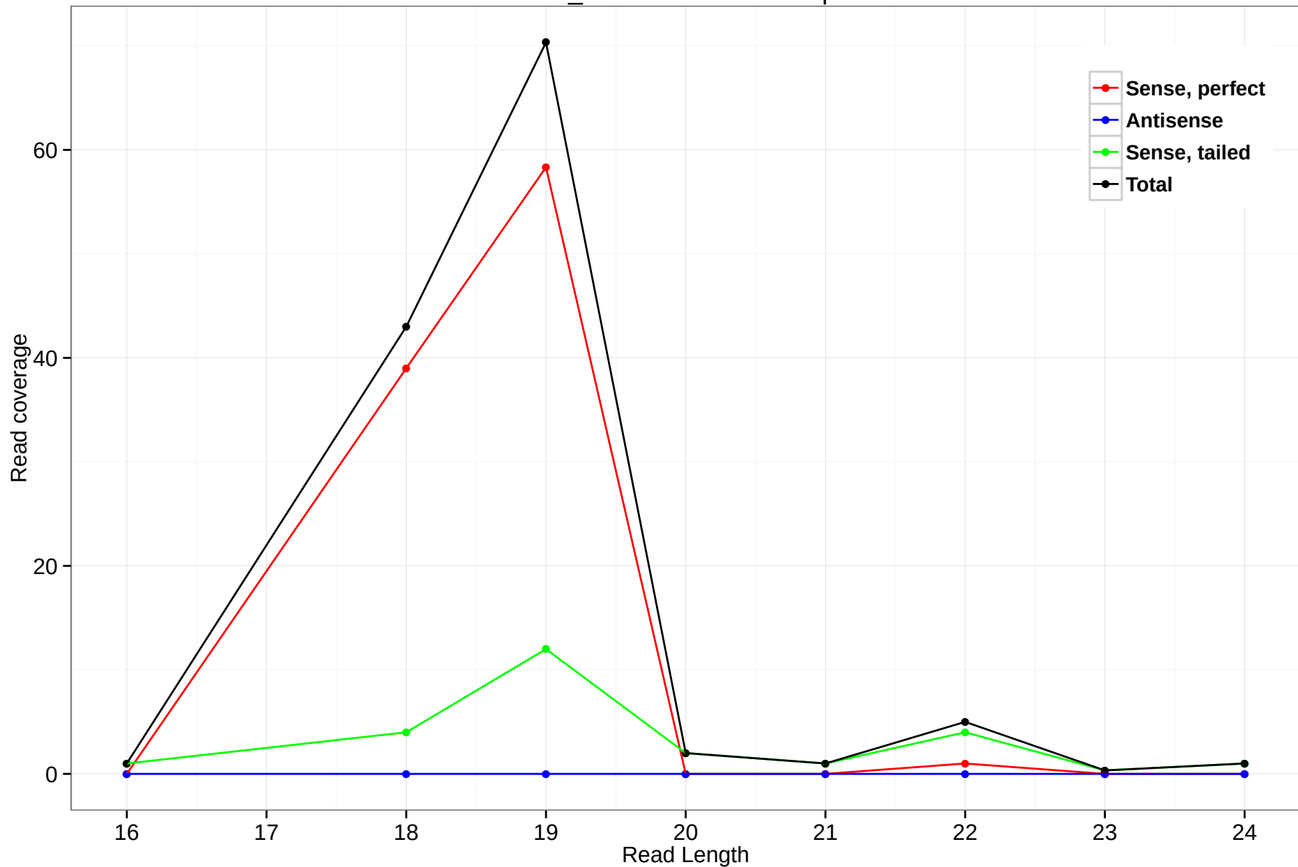
2R_8186118-8191201.5p
