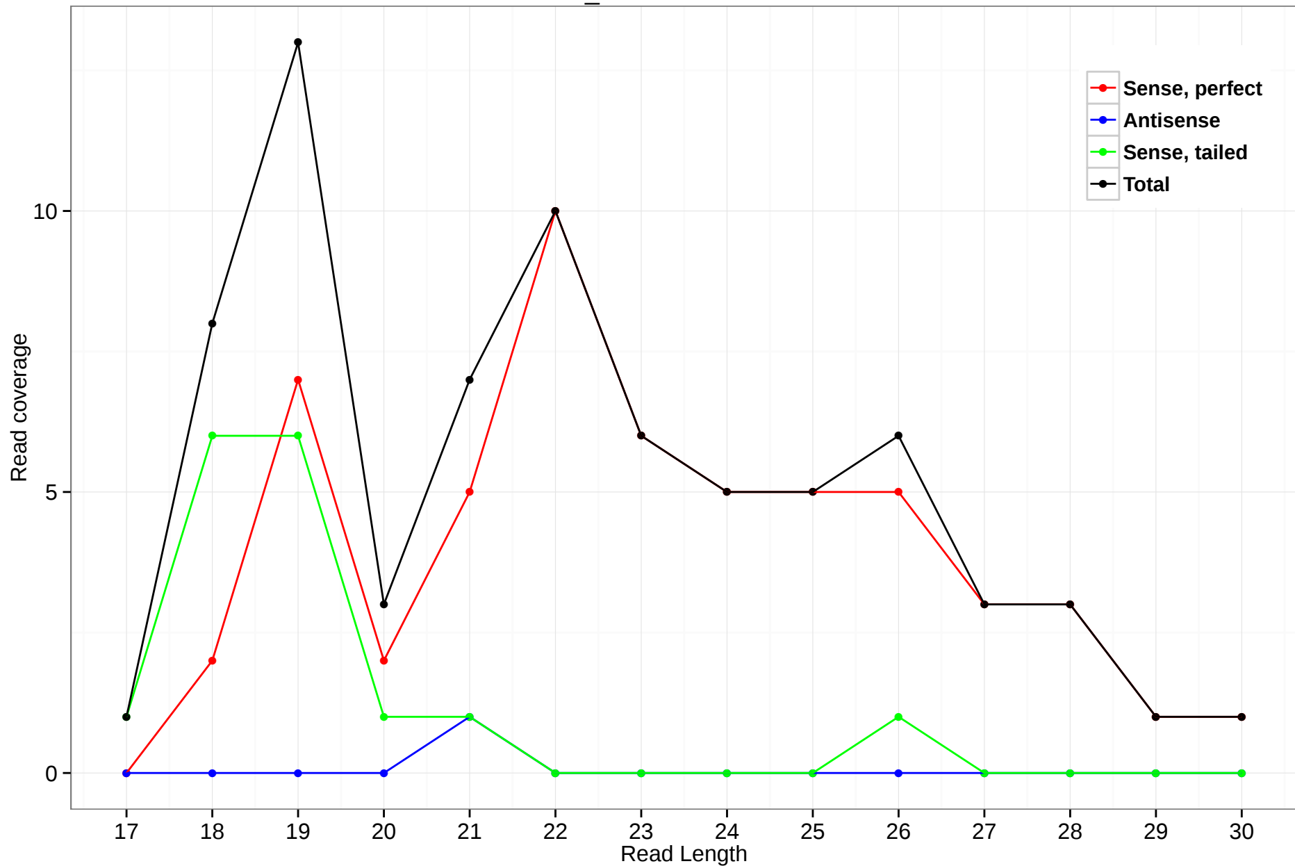
2R_4375315-4375560
