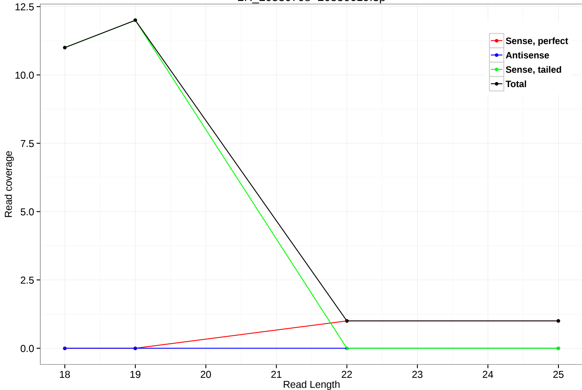
2R_20530768-20536619.3p
