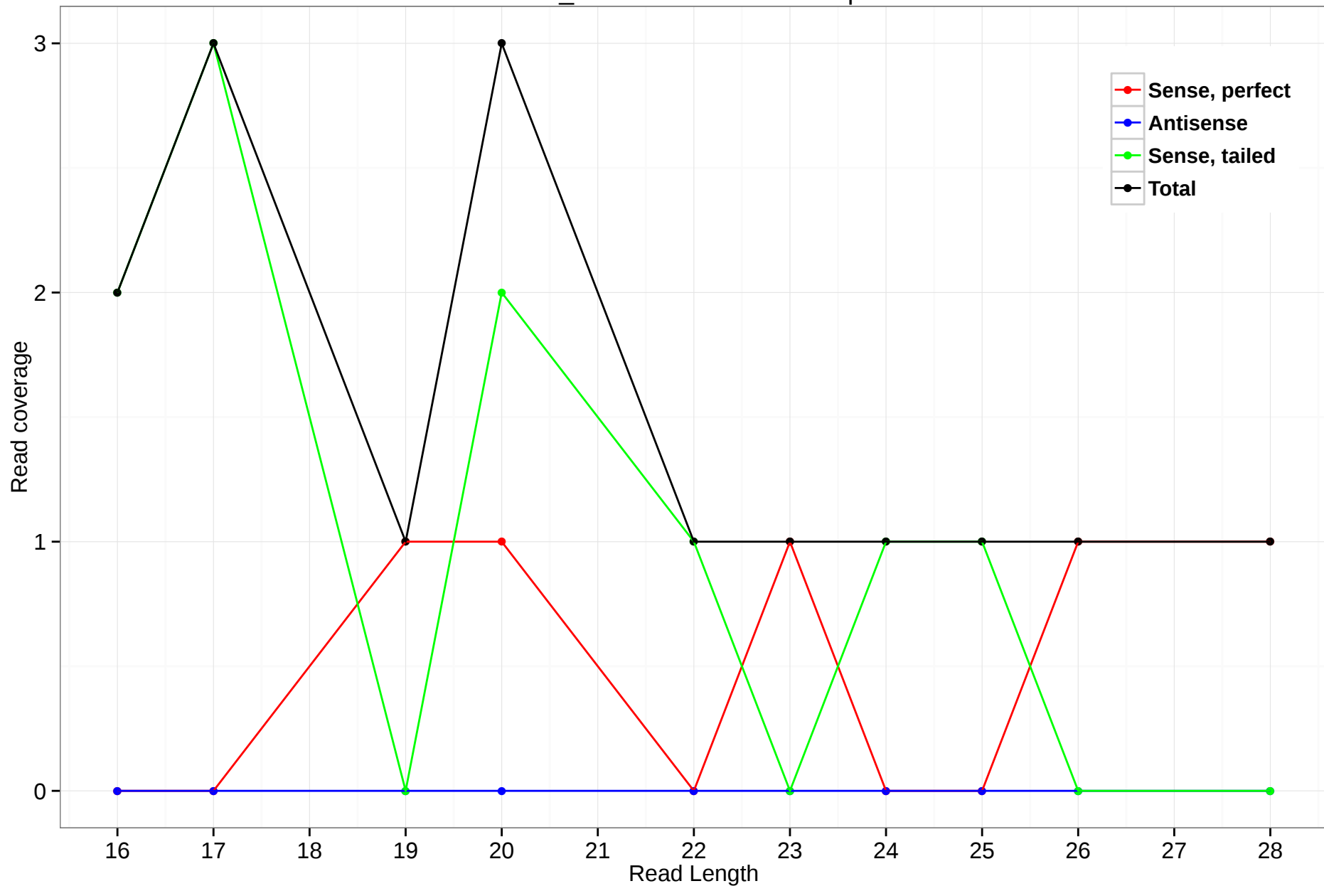
2R_20151018-20151436.3p
