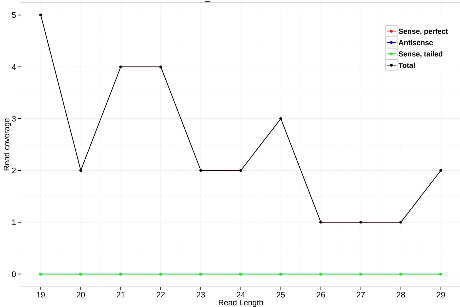
2L_6263514-6263818
