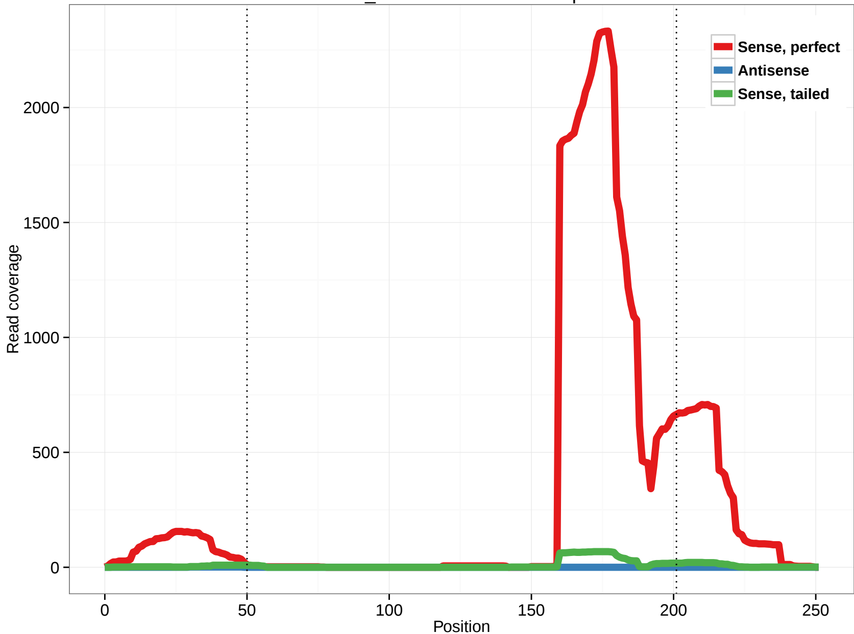
3R_11081104-11081858.5p
