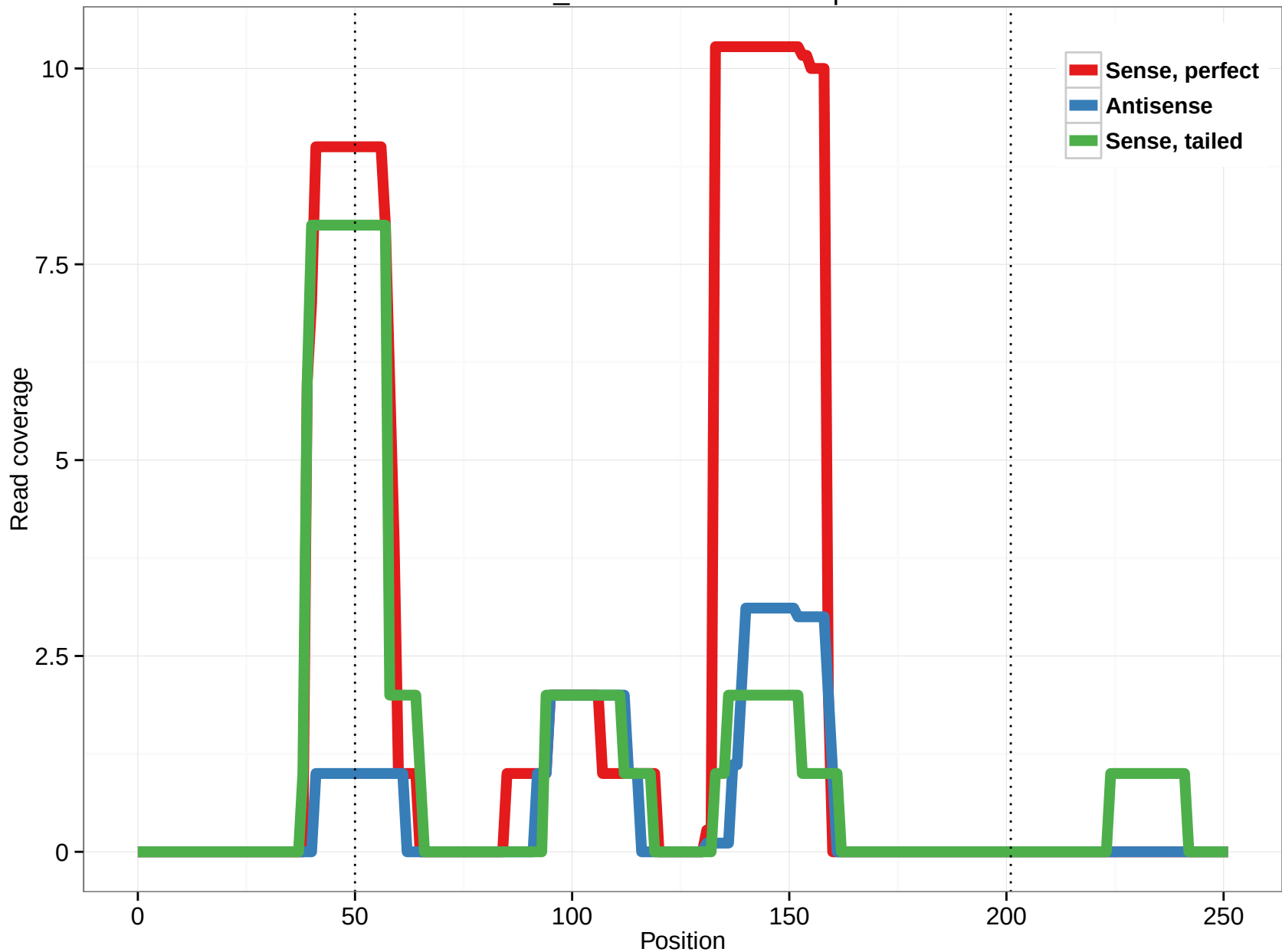
2R_1126753-1127231.3p
