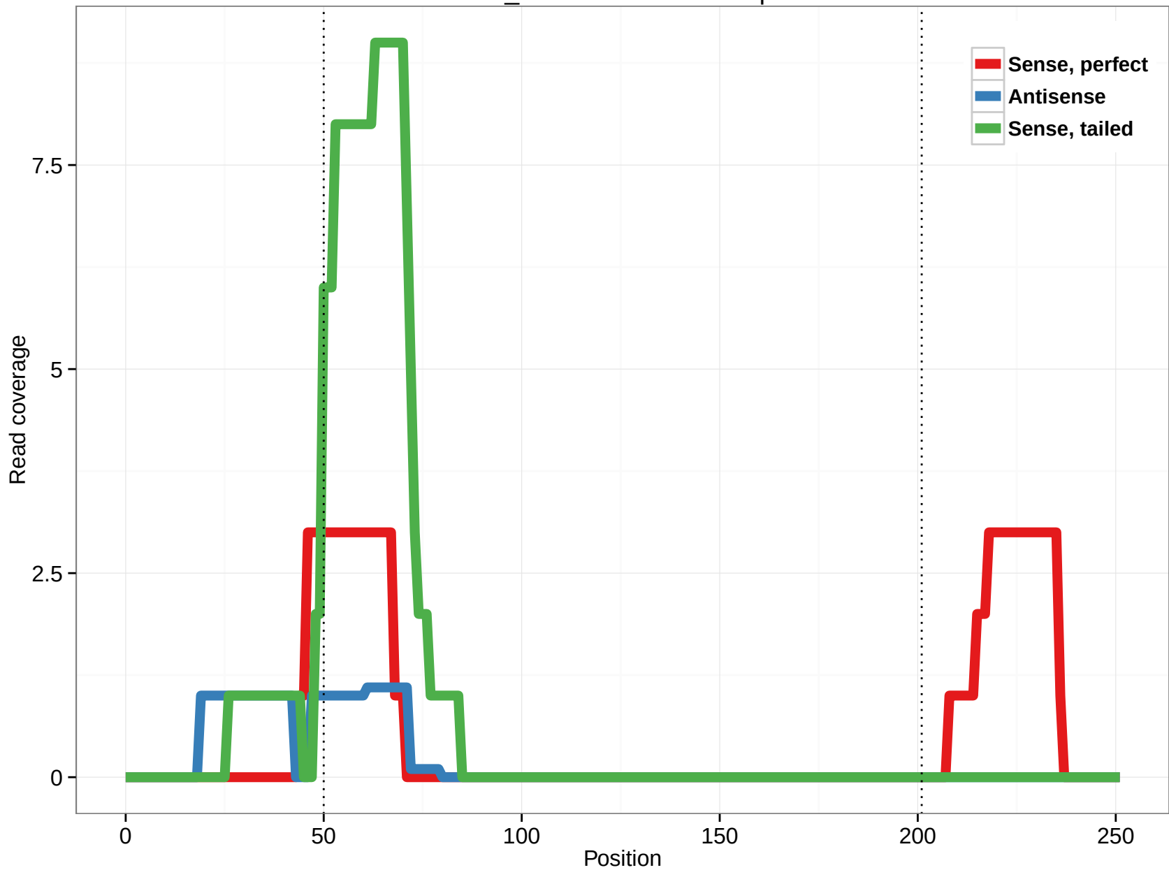
2R_1101910-1108714.3p
